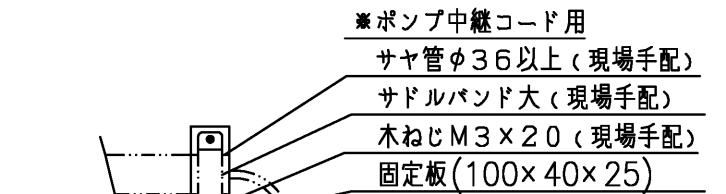
サヤ管固定部詳細図
